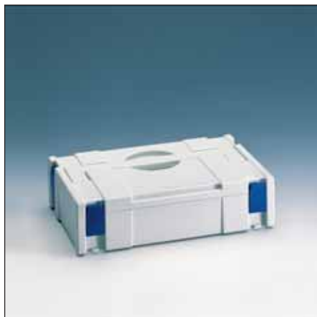
MINI-systainer® I outside dimensions H 70 x W 268 x D 171 mm light grey art n° 559-040 anthracite art n° 559-033
